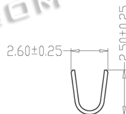
SEC:B-B
