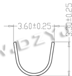
SEC:A-A
